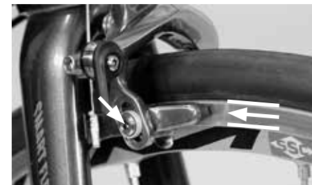
ブレーキシューはリムとぴったり方向が合っていないといけません
