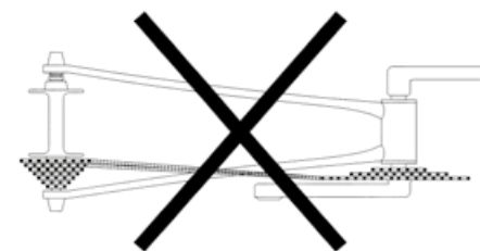
悪いチェーンの掛かり方 — 前が一番大きなチェーンリングで後ろが一番大きいスプロケット
