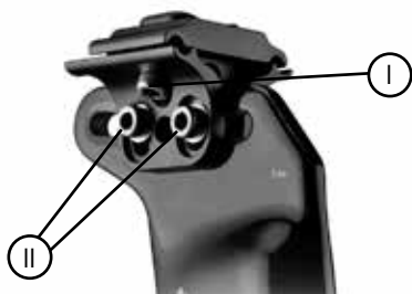
Speedmax のサドルクランプについての固定用と調整用の六角穴ボルト
