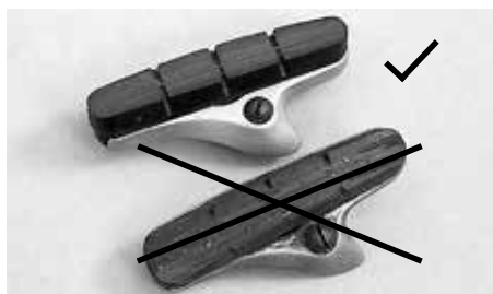
Calços dos travões, nos quais as ranhuras (indicadores de desgaste) estão gastas (em baixo), têm que ser substituídos por calços sobresselentes de origem
