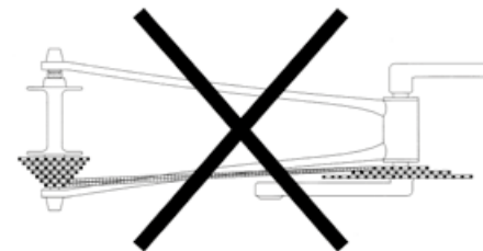
Incorreto andamento da corrente – corrente engata no prato menor à frente, e no pinhão menor atrás
