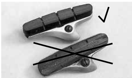
Calços dos travões, nos quais as ranhuras (indicadores de desgaste) estão gastas (em baixo), têm que ser substituídos
