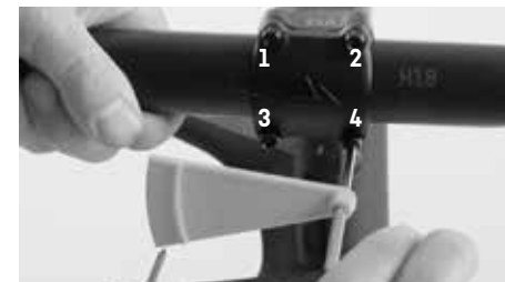
Aperte bem os parafusos consoante o torque marcado
