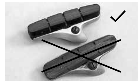
Okładziny hamulców, w których rowki (wskaźniki zużycia) są zdarte (dolna), trzeba wymienić na oryginalne części zamienne
