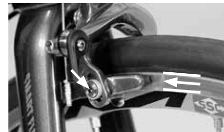
Okładzina hamulcowa musi dokładnie trafić w obręcz
